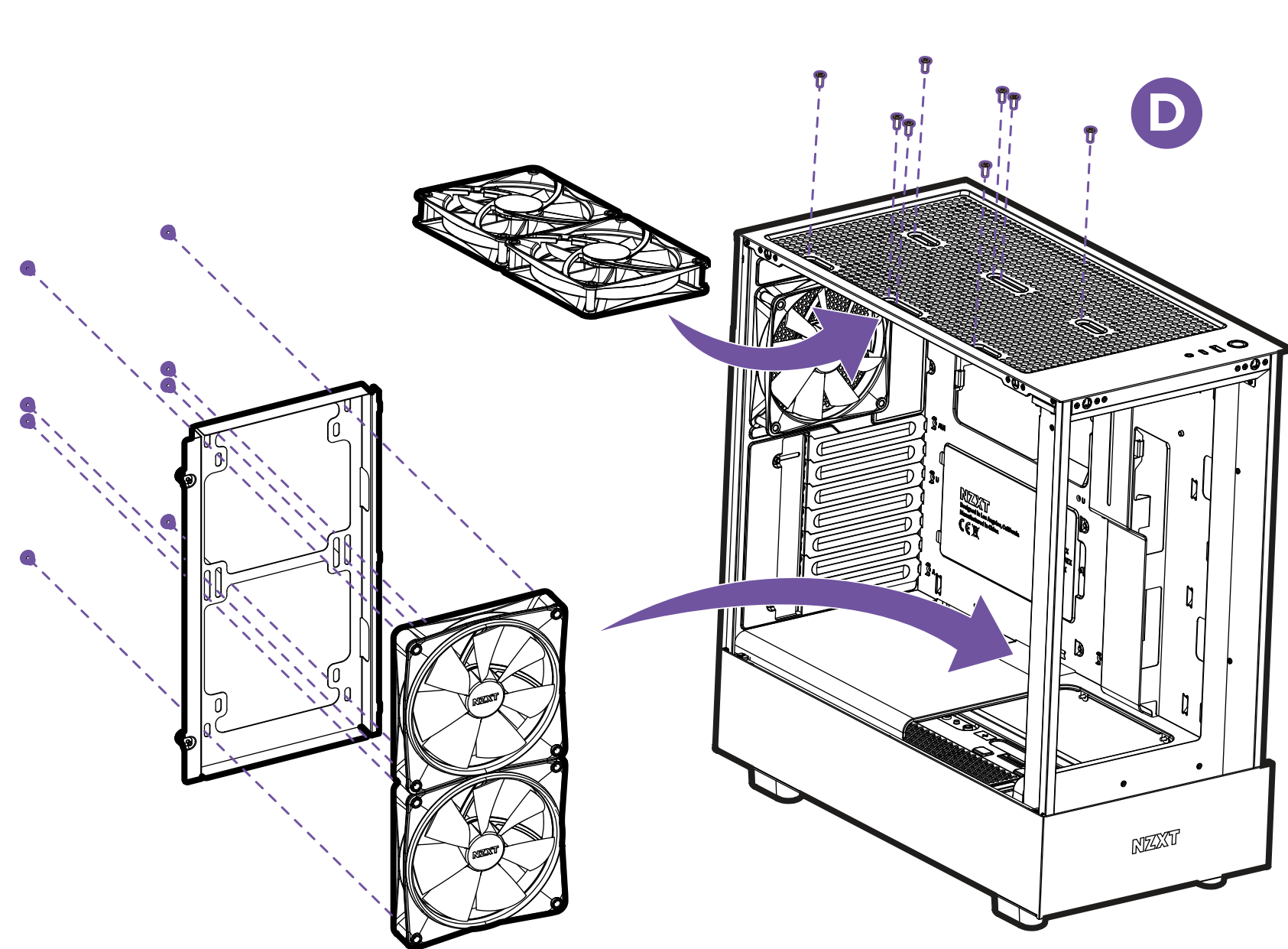
VENTILATEUR
